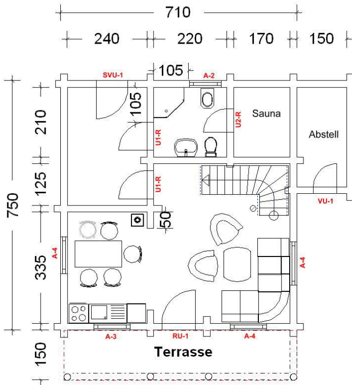
Erdgeschoss
