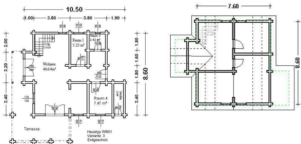
Variante 3 (ca. 90 qm)
